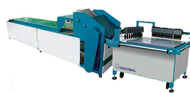
Mały stół do rozkroju szkła Cutting & Breaking machine
