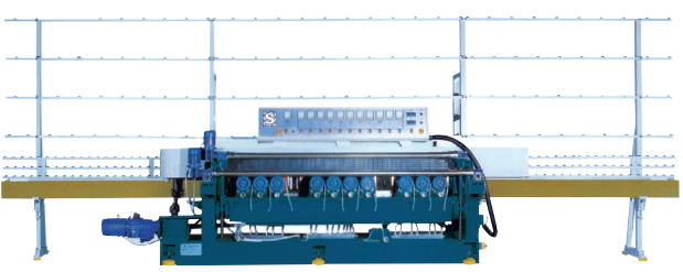
Fazowarka 11 głowicowa Motors glass beveling machine
